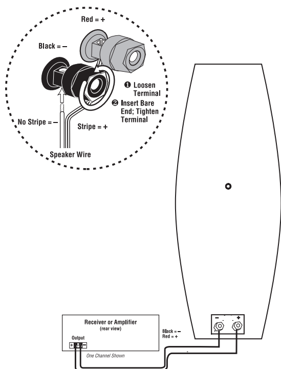
Figur 3. Kopplingsdiagram visar polaritetskopplingar för en kanal i ett hemmabiosystem.
