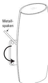
Figur 2. Monteringsjärn på väggen.
